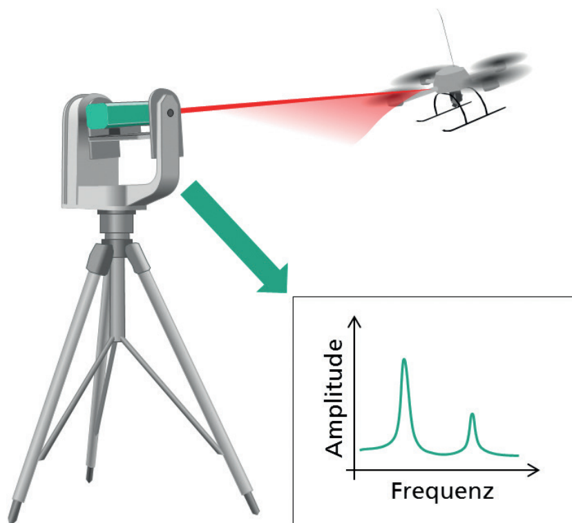
Abb. 3: Einsatz eines Laser-Vibrometers zur Unterstützung bei der Drohnenaufklärung.
